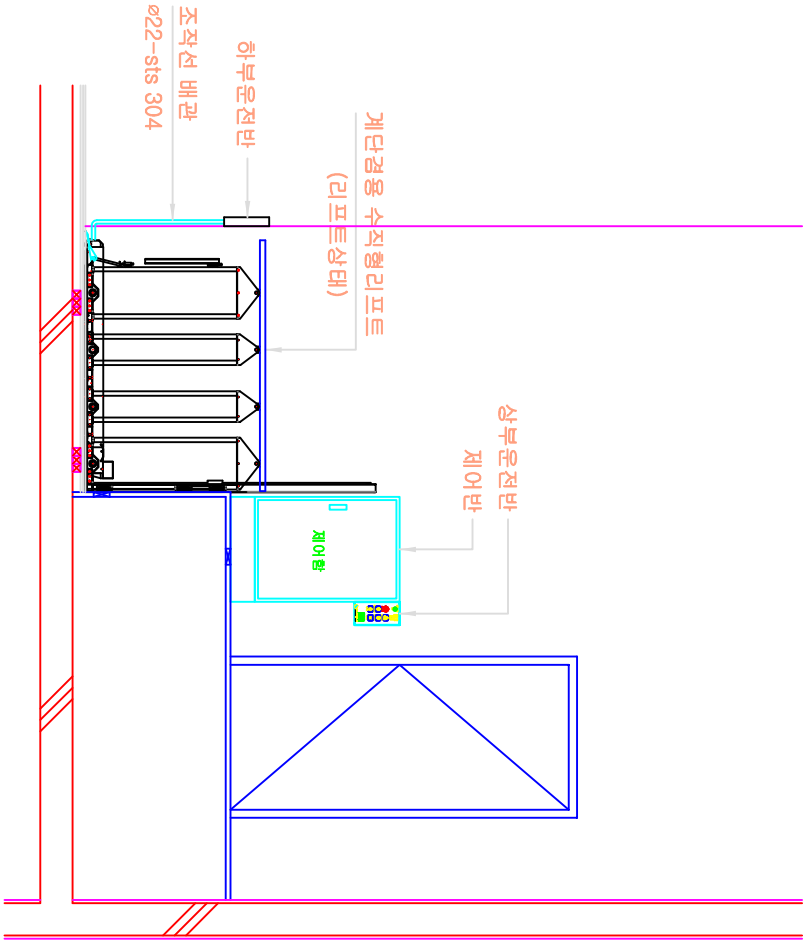
설치 단면도(리프트 상태)
