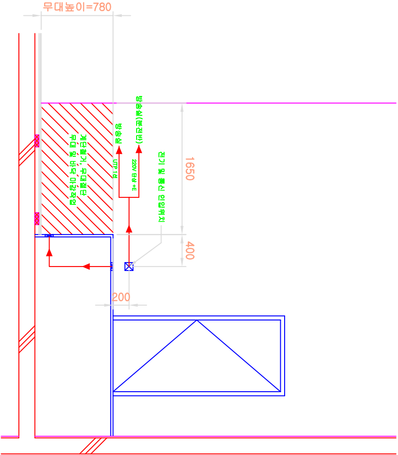
부대공사 단면(변경 후)
